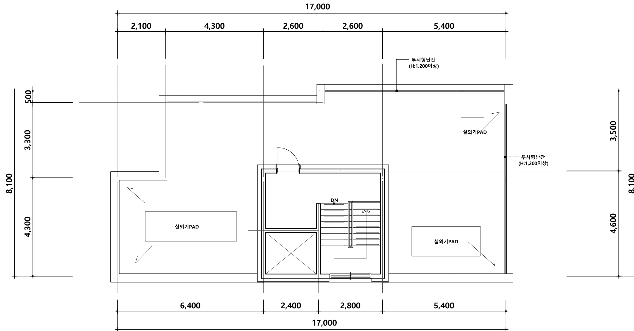
옥탑 1층 평면도
